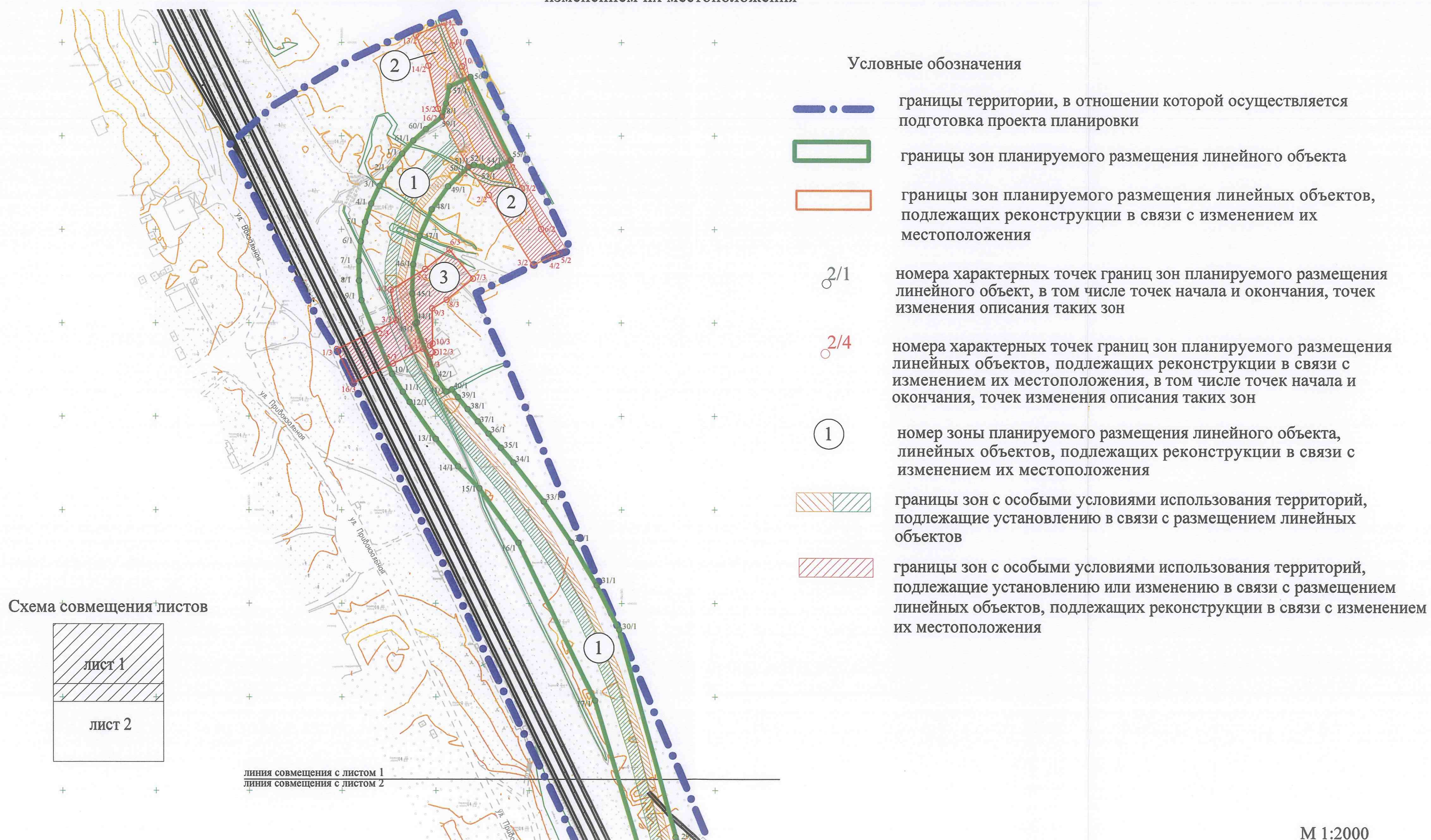
Чертеж границ зон планируемого размещения линейного объекта, чертеж границ зон планируемого размещения линейных объектов, подлежащих реконструкции в связи с изменением их местоположения
