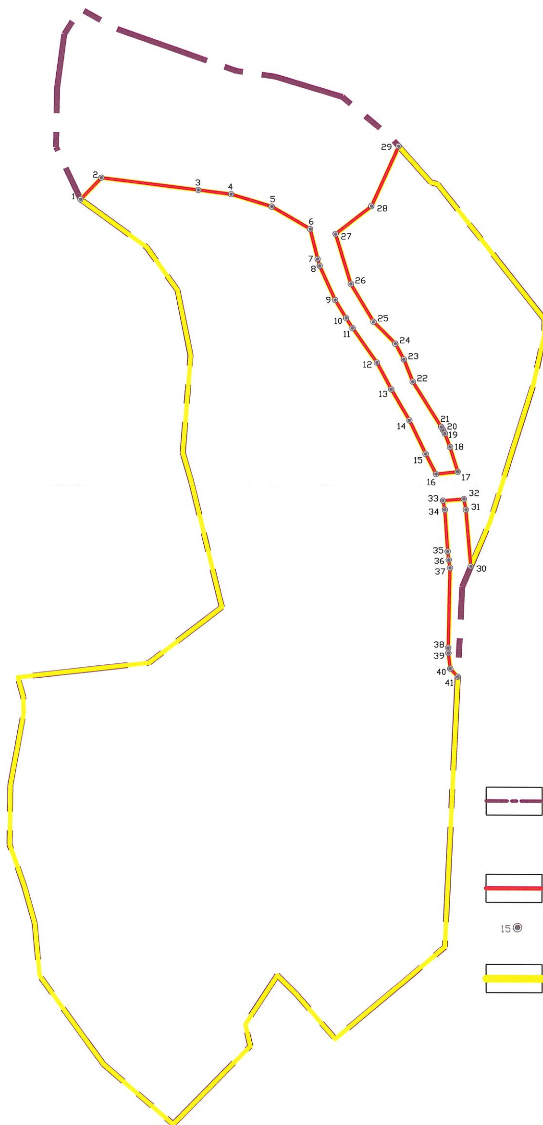
Чертеж планировки территории, отображающий красные линии, границы планируемых элементов планировочной структуры
